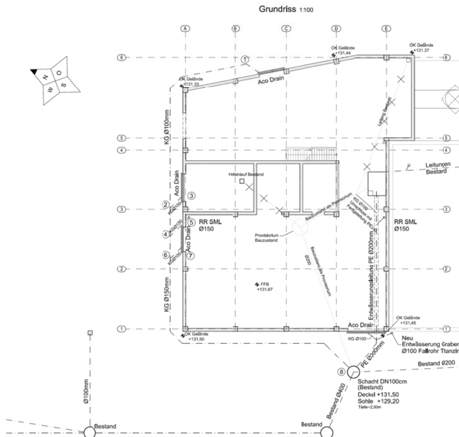
Vista plana del sistema de agua residual del edificio de calderas © rmd-consult
